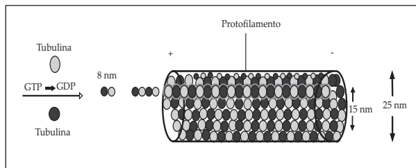
Figura 1. Esquema simplificado que ilustra los pasos en el ensamblaje de un microtúbulo.
